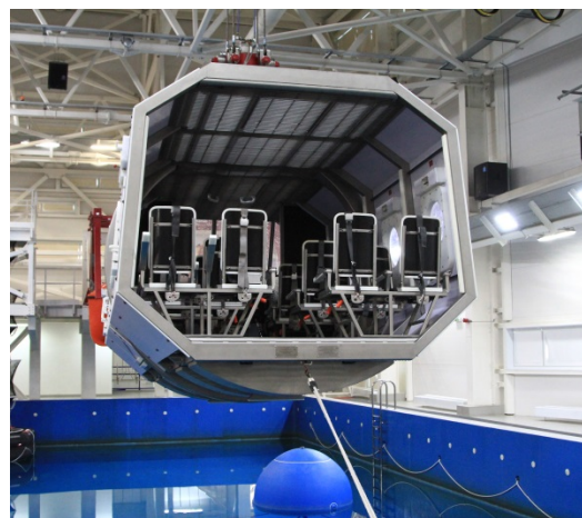
Рисунок 2 – Общий вид салона погружного макета вертолета
